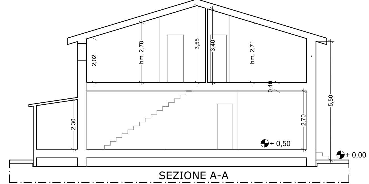
SEZIONE A-A
