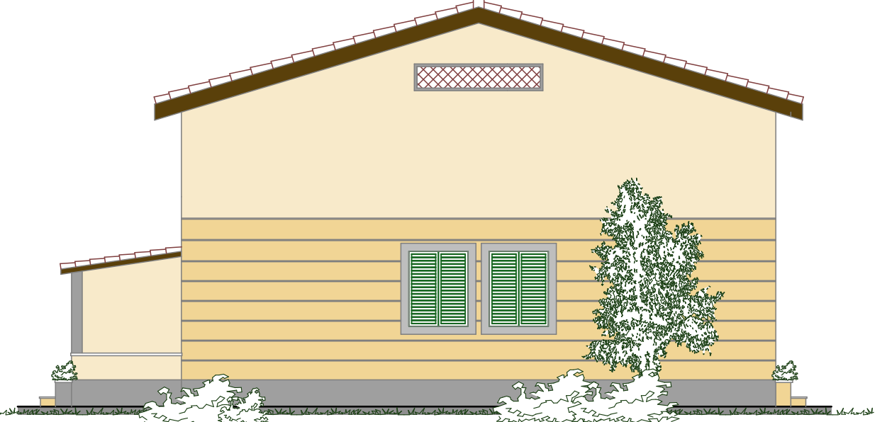
PROSPETTO NORD
